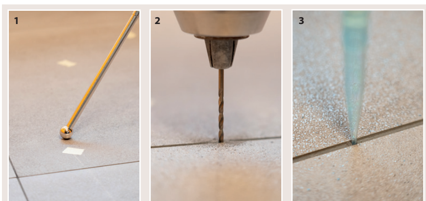
Etapy naprawy okładziny ceramicznej w przypadku występowania pustych przestrzeni pod płytkami: 1. zlokalizowanie pustej przestrzeni dedykowanym wykrywaczem; 2. wywiercenie otworu 2 mm; 3. wypełnienie pustych przestrzeni preparatem Gap Filler przez wywiercony otwór
