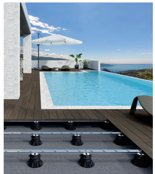
Fot. 6. Przykład rozwiązania systemowego ETERNO IVICA z użyciem aluminiowych legarów
