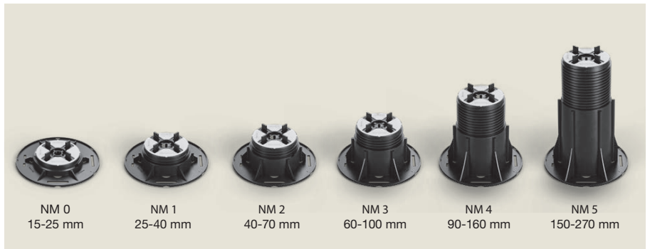
Fot. 4. Jedna z serii podpór regulowanych New Maxi z głowicą tworzywowo-gumową
