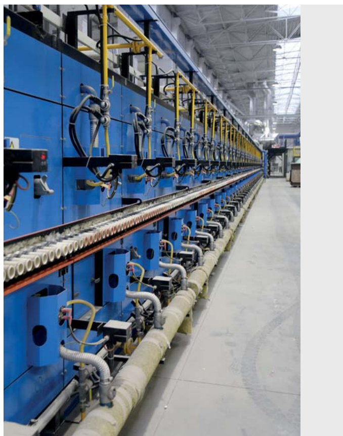
Piec do wypalania płytek (o długości 124 m) firmy SACMI
